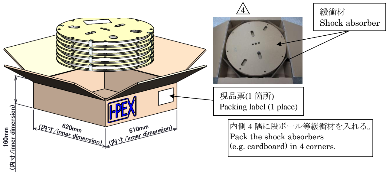
① 図 2. 外箱梱包 / Fig. 2. Packing of carton
