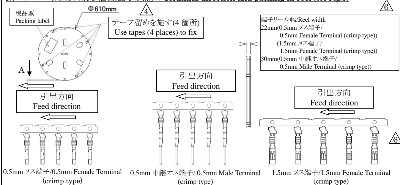
図1. リールへの梱包 / Fig.1. Packing in reel
