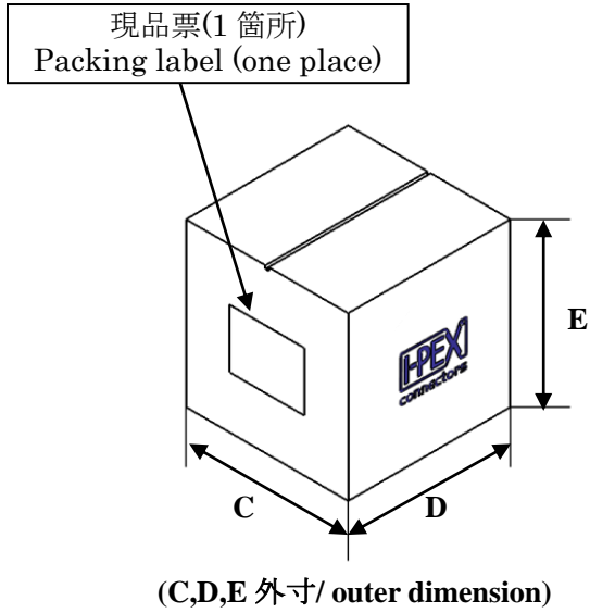
図 3.外箱仕様 Fig3. Packing carton box specification
