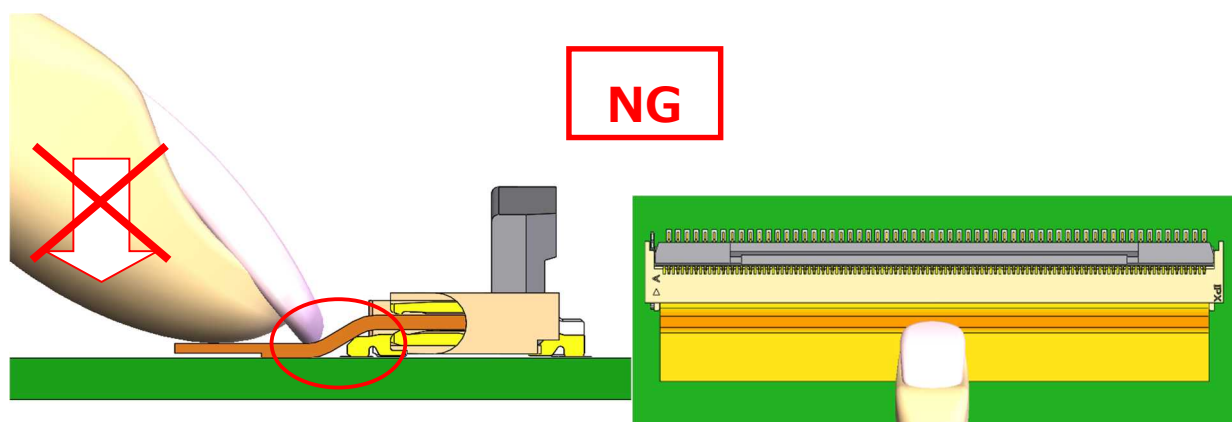
図 10. FPC 挿入方法 (NG) / Fig.10 FPC insertion (NG)
