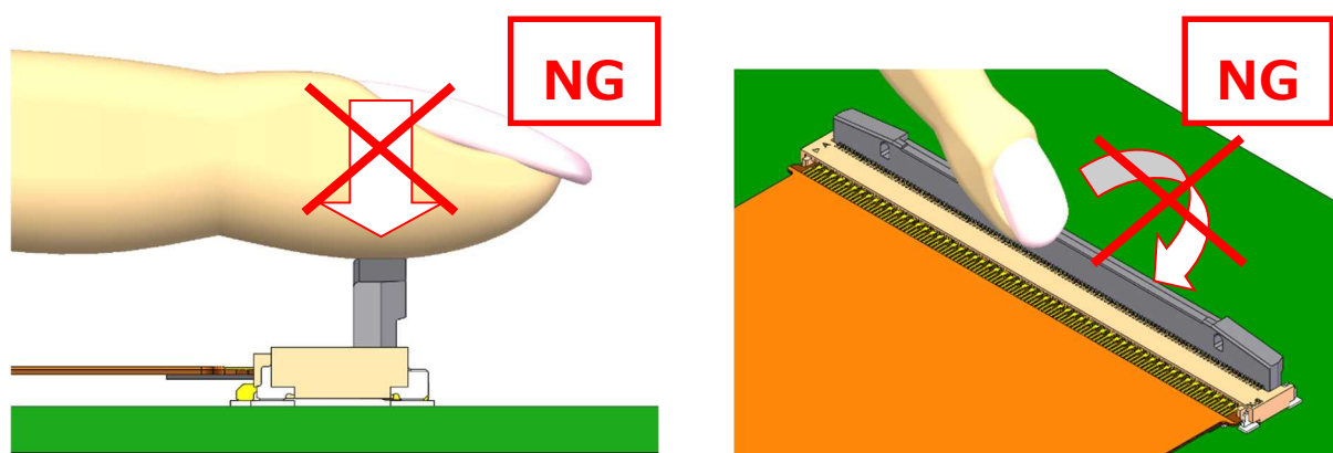
図 12. アクチュエータのロック方法 (NG) / Fig.12 To lock actuator (NG)
