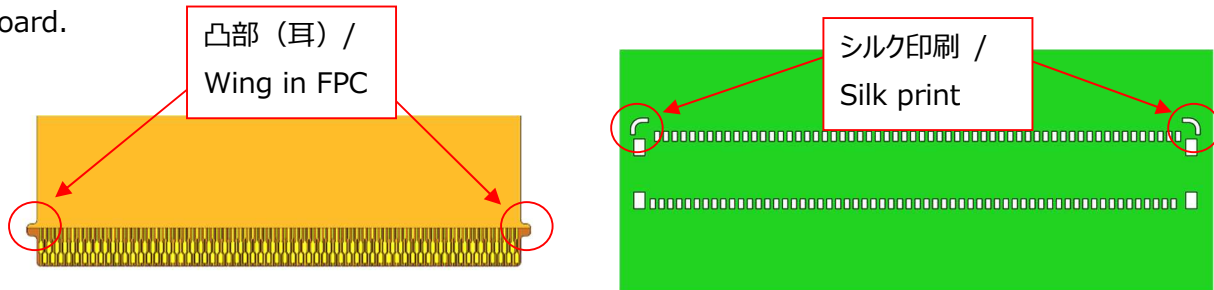
図 6. FPC の挿入確認用（参考） / Fig.6 The check of FPC insertion (Reference)
