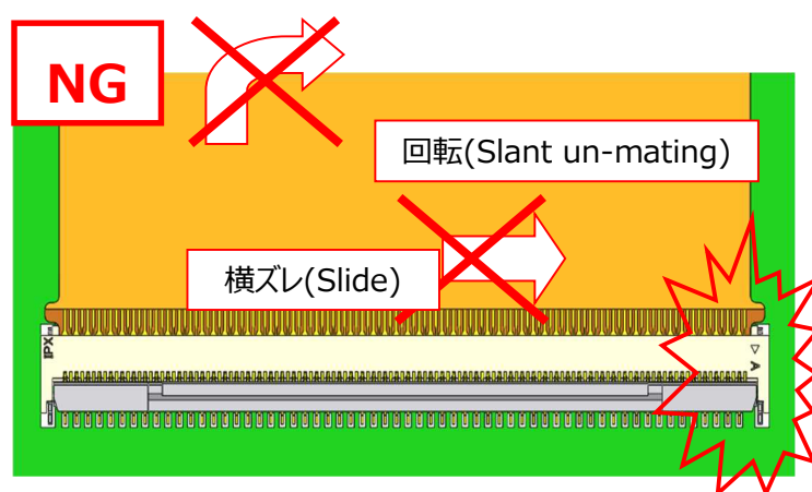
図 9. FPC 挿入方法 (NG) / Fig.9 FPC insertion (NG)
