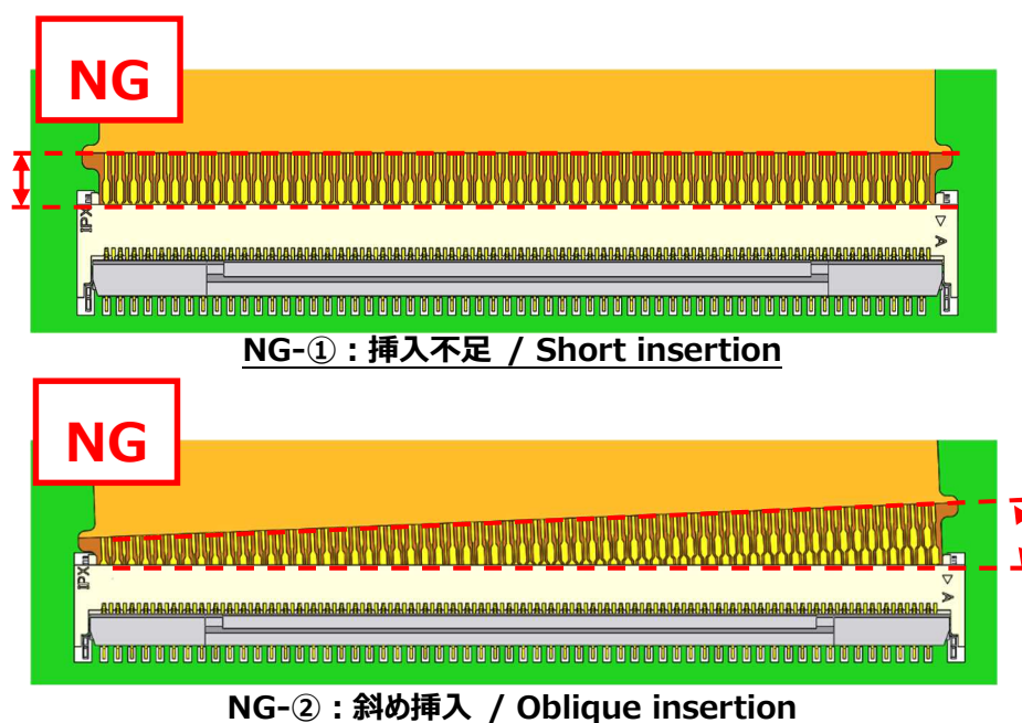
図 5. FPC 挿入方法 (NG) / Fig.5 FPC insertion (NG)
