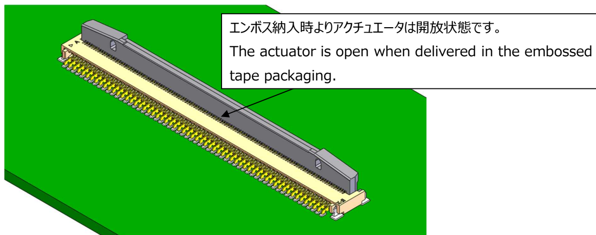
図 2. コネクタ実装状態 / Fig.2 Connector mounting state
