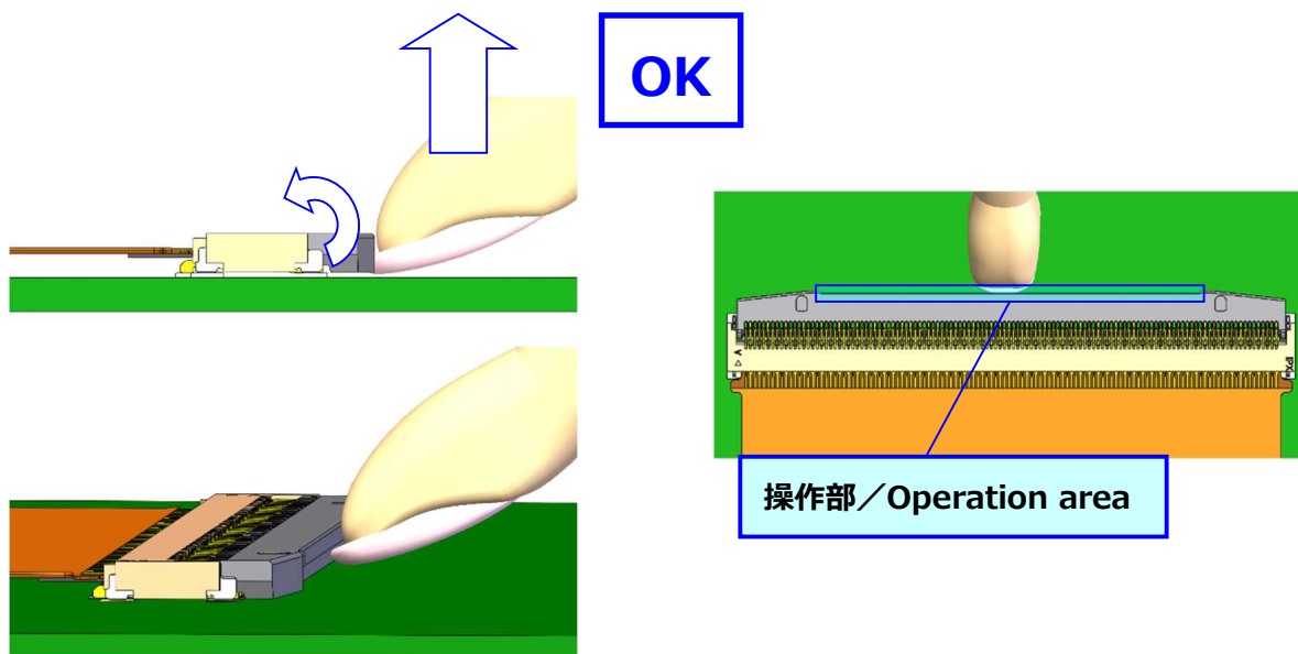
図 16. アクチュエータの解除方法 (OK) / Fig.16 To release actuator (OK)
