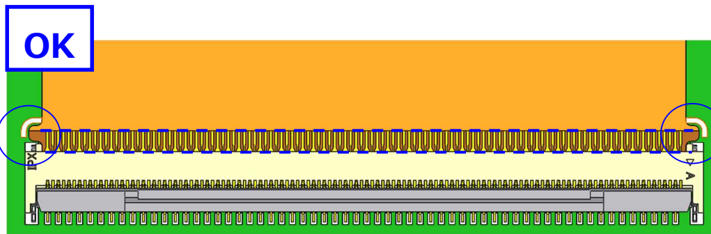
図 6. FPC の挿入確認用（参考） / Fig.6 The check of FPC insertion (Reference)
