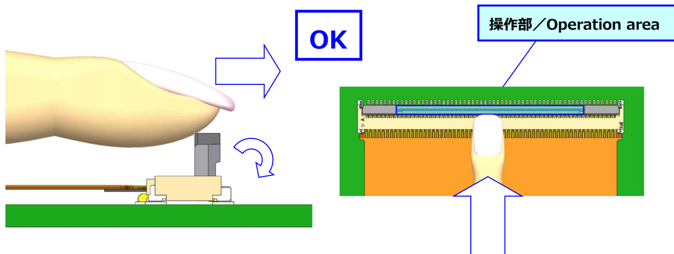
図 11. アクチュエータのロック方法 (OK) / Fig.11 To lock actuator (OK)
