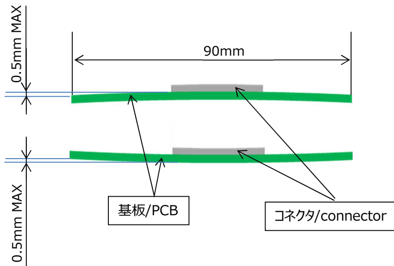
図 21. 基板反り量 / Fig.21 Amount of PCB warp
