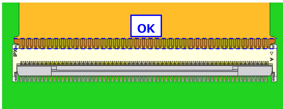
図 4. FPC 挿入方法 (OK) / Fig.4 FPC insertion (OK)
