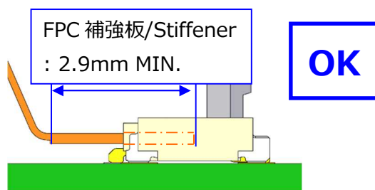
図 19 FPC の屈曲 (OK) / Fig.19 Flexion of FPC (OK)
