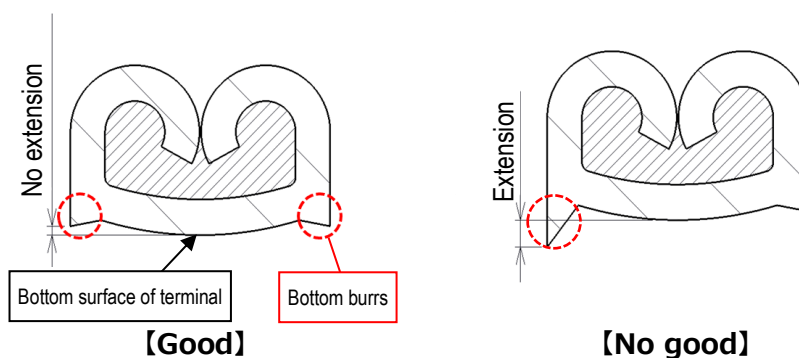
Fig 11. Bottom burrs
