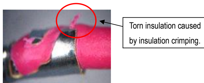
Fig 25. Torn insulation
