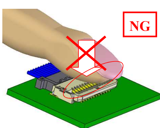
図 10 アクチュエータのロック方法 (NG) / Fig.10 To lock actuator (NG)
