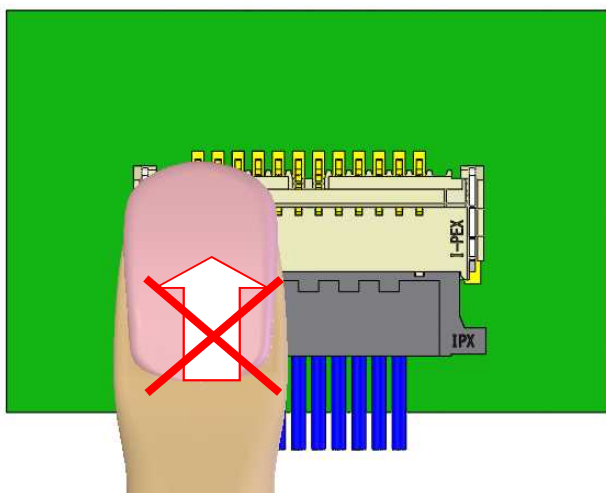
図 9 アクチュエータのロック方法 (NG) / Fig.9 To lock actuator (NG)
