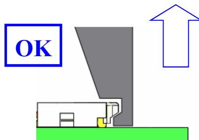
図 12 アクチュエータの解除方法 (OK) / Fig.12 To release actuator (OK)
