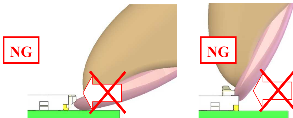
図 13 アクチュエータの解除方法 (NG) / Fig.13 To release actuator (NG)
