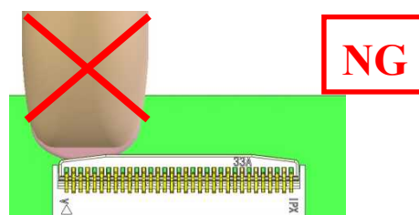
図 14 アクチュエータのロック方法 (NG) / Fig.14 To lock actuator (NG)
