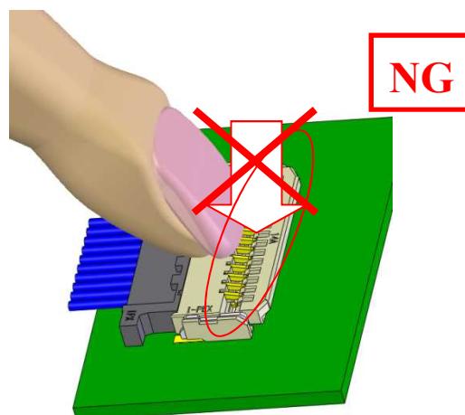
図 10 アクチュエータのロック方法 (NG) / Fig.10 To lock actuator (NG)
